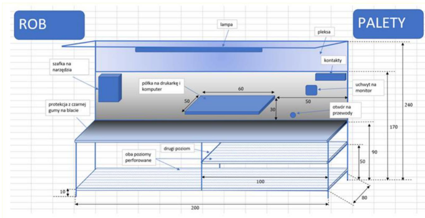
Rys. 1 – Przykładowy widok stanowiska do pakowania
