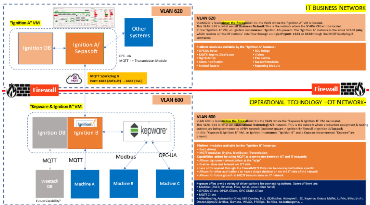
Rys.7. Propozycja architektury
