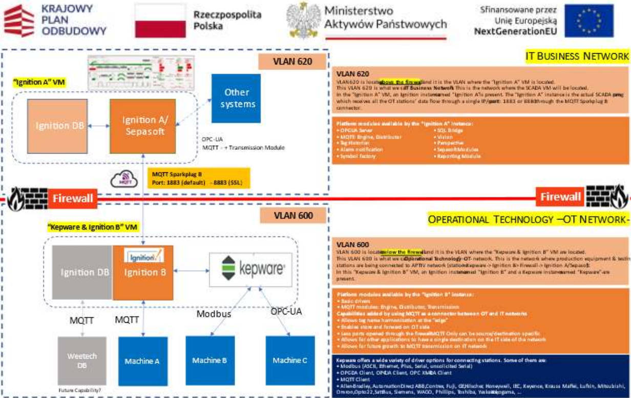
Rys.7. Propozycja architektury
